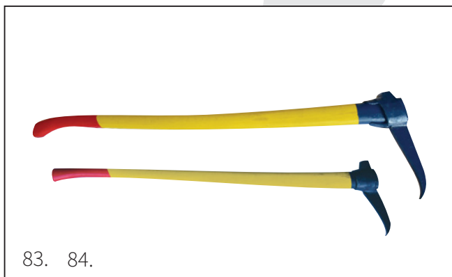
Cepin 1,00/ 1,80 kg
